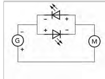
Taschenlampe Schaltplan A
