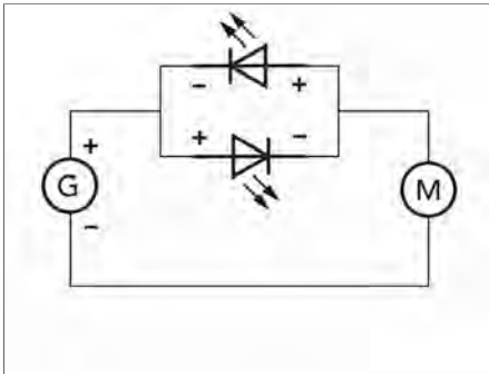
Taschenlampe Schaltplan B
